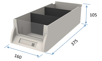
ART NO: HD-18 S/G/E Bin QTY ← S - Steel door G - Glass door E - Without door
