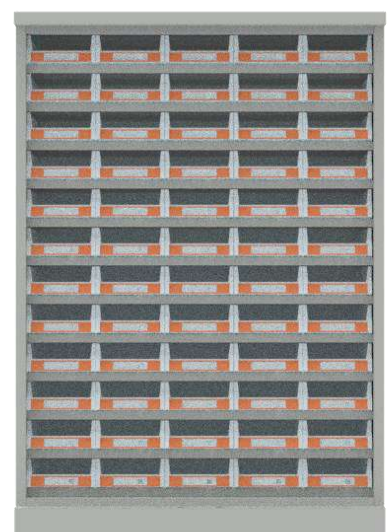
ART NO: LD-60 E 880W x 376D x 1248H
